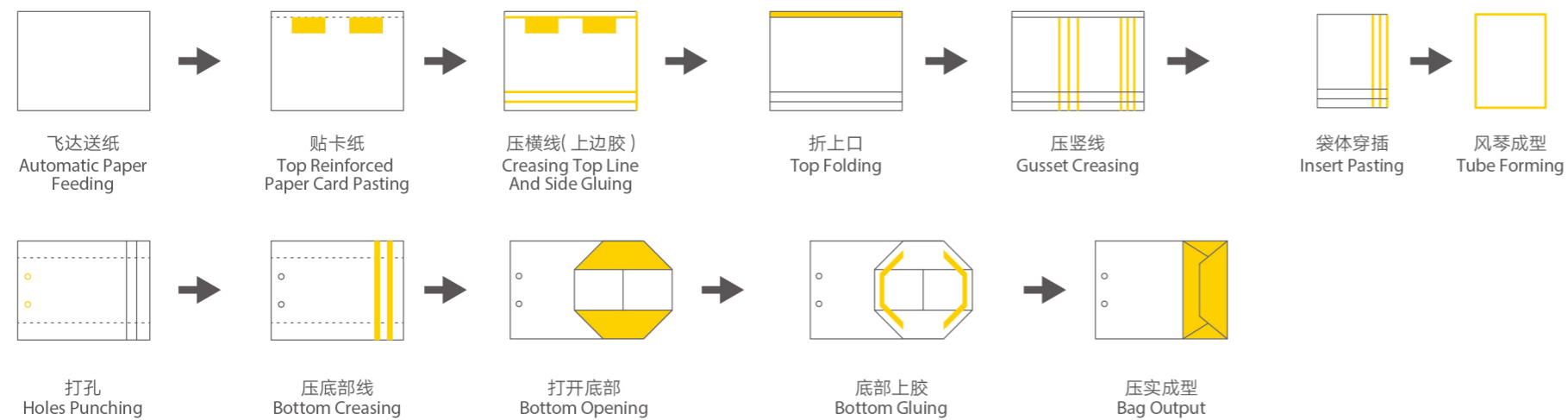
工艺流程图 Process flowa
