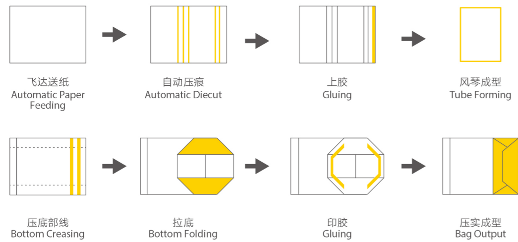
工艺流程图 Process flow
